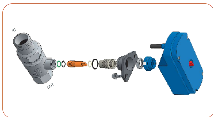
Esplodo valvola a sfera con attuatore elettrico Exploded view drawing of electro-motor actuated ball valve
